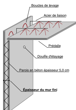
Murs précoffrés
